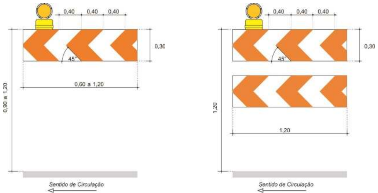
Barreira Tipo I
